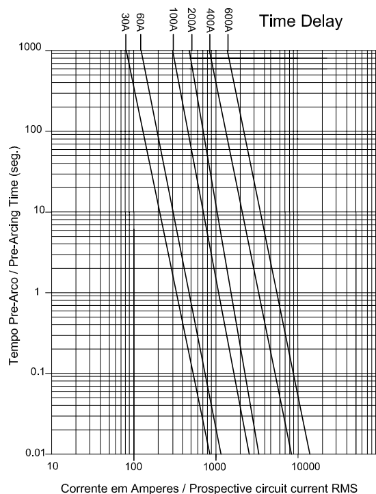
Tempo Corrente / Time - Current Curve
