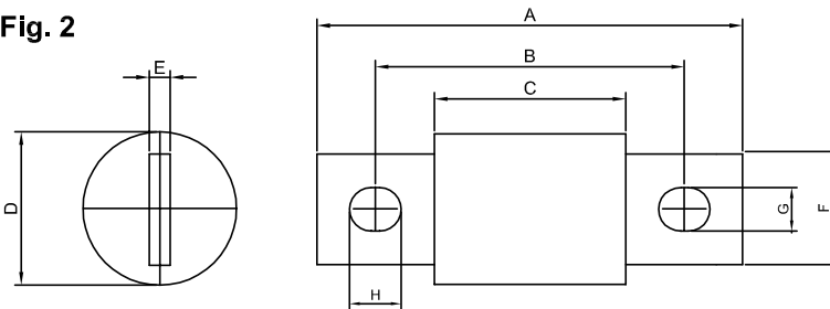
Dimensões / Dimensions (mm in parentheses)
