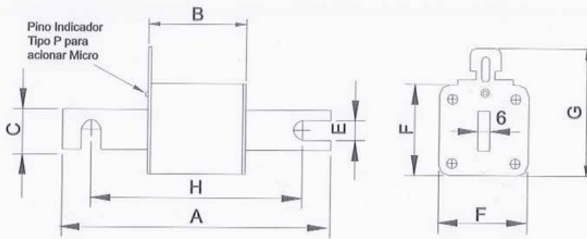
Fig. 2 - DIN 43653 Tam. 1,2,3 - Standard Alemão / German Standard
