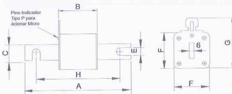
Fig. 2 - DIN 43653 Tam.1,2,3 - Standard Alemão / German Standard
