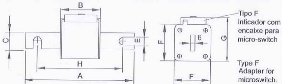
Fig. 2 - DIN 43653 Tam.1,2,3 - Standard Alemão / German Standard
